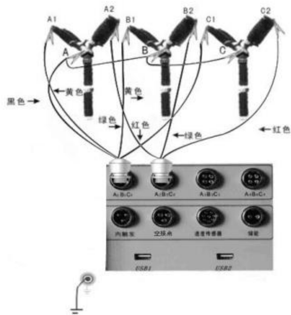
断口接线图（六断口）
