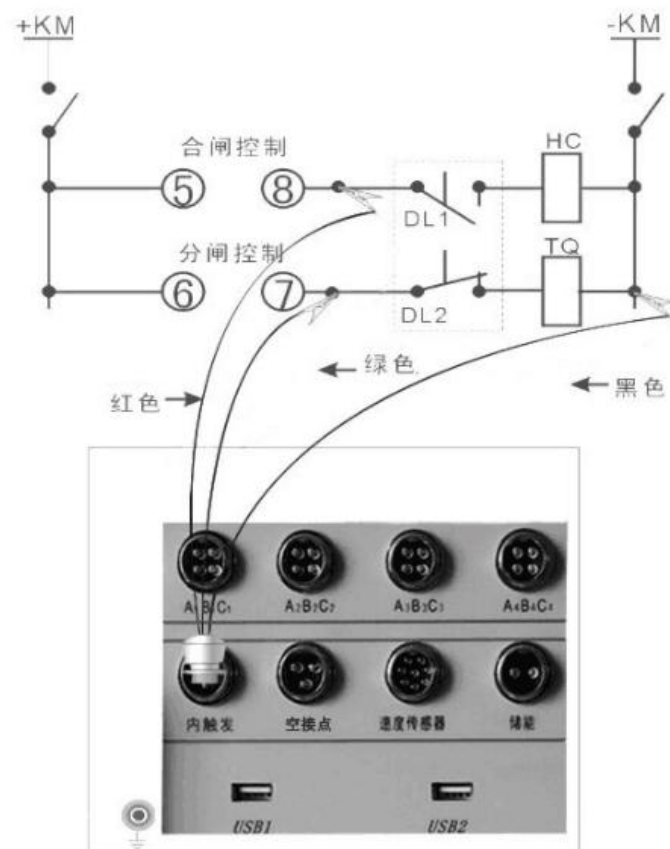
高压开关控制屏内触发控制接线示意图
