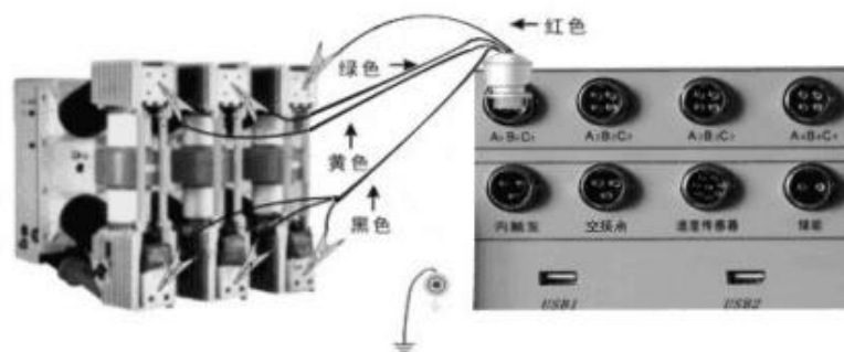
断口接线图（六断口）
