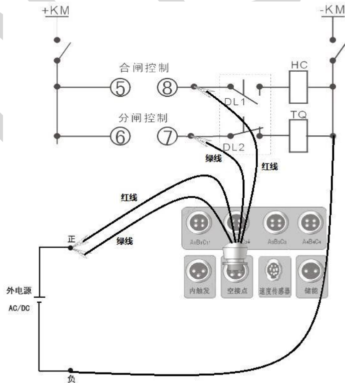
高压开关控制屏空接点控制接线示意图
